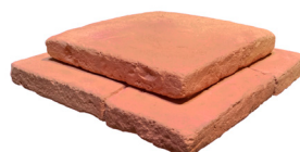
Chapeau de pilier BRIQUE (avec goutte d'eau) L. 45 x l. 45 x H. 11 cm
